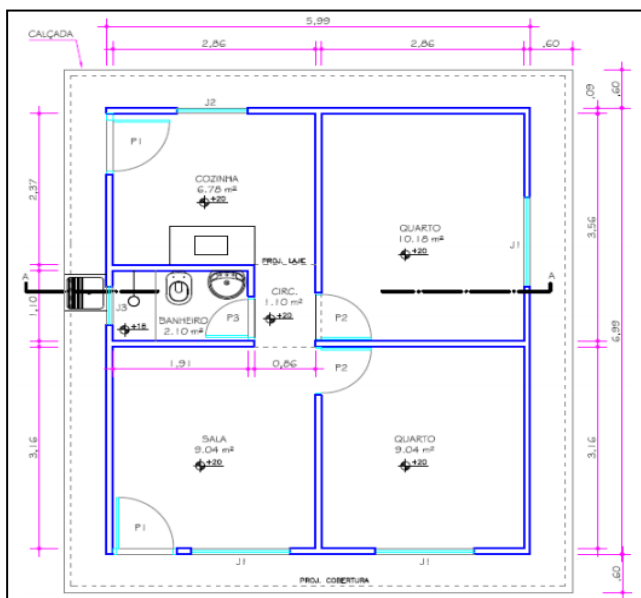
Figura 2: Planta baixa do projeto original.
