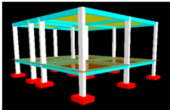
Figura 3: Esquema de pórtico em 3D da estrutura no Eberick.
