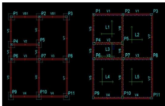
Figura 4: Planta estrutural de fundação e térreo, respectivamente.
